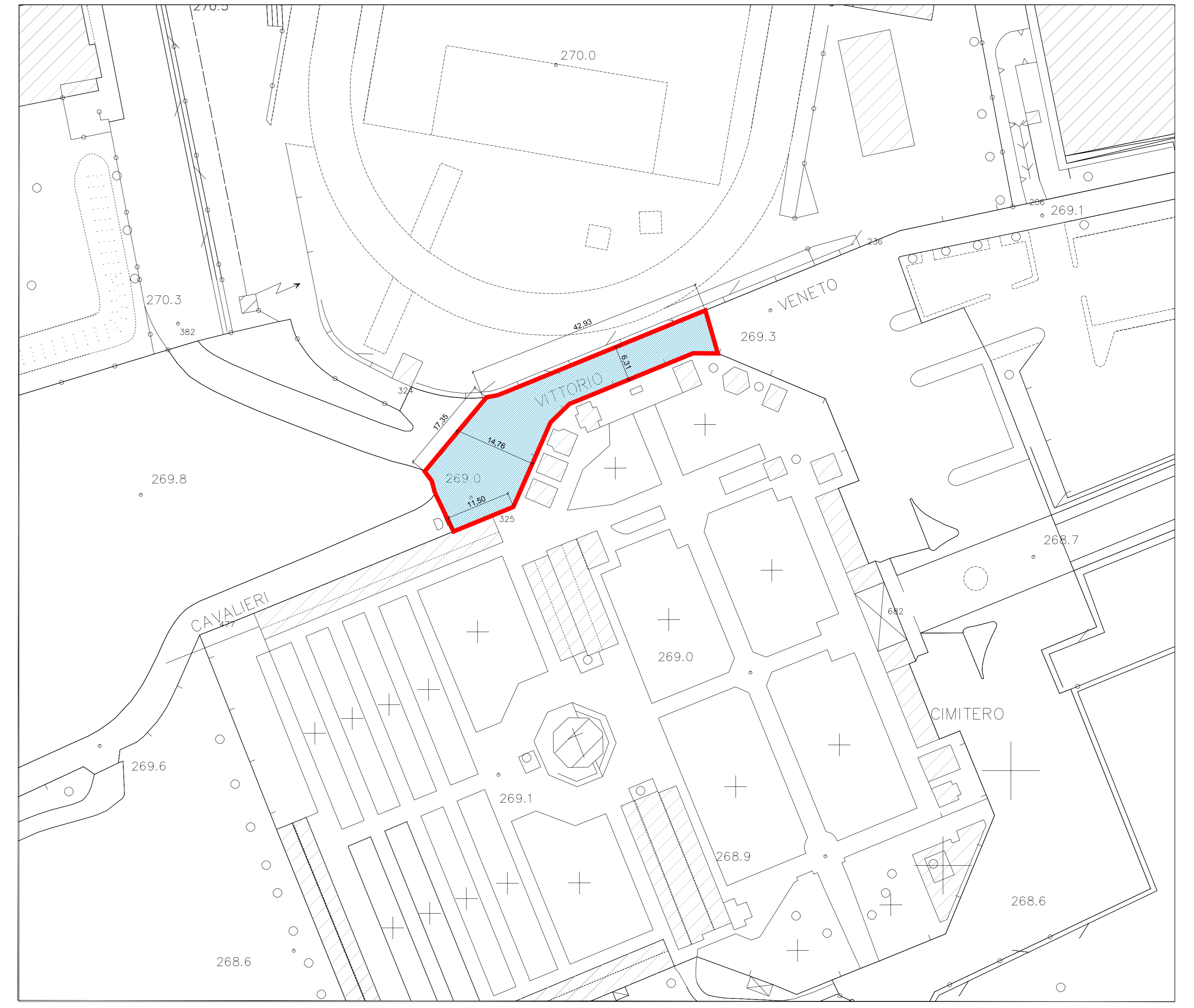
PROGETTO - PLANIMETRIA VIA CAVALIERI DI VITTORIO VENETO - SCALA 1:500
