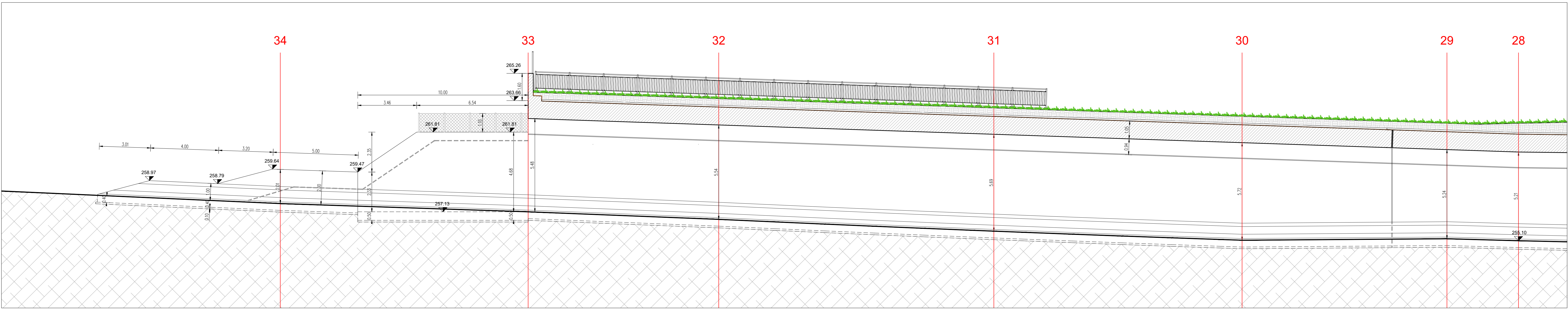
SEZIONE/PROSPETTO A_A - VISTA SUD - LATO SOLZA - Scala 1:100
