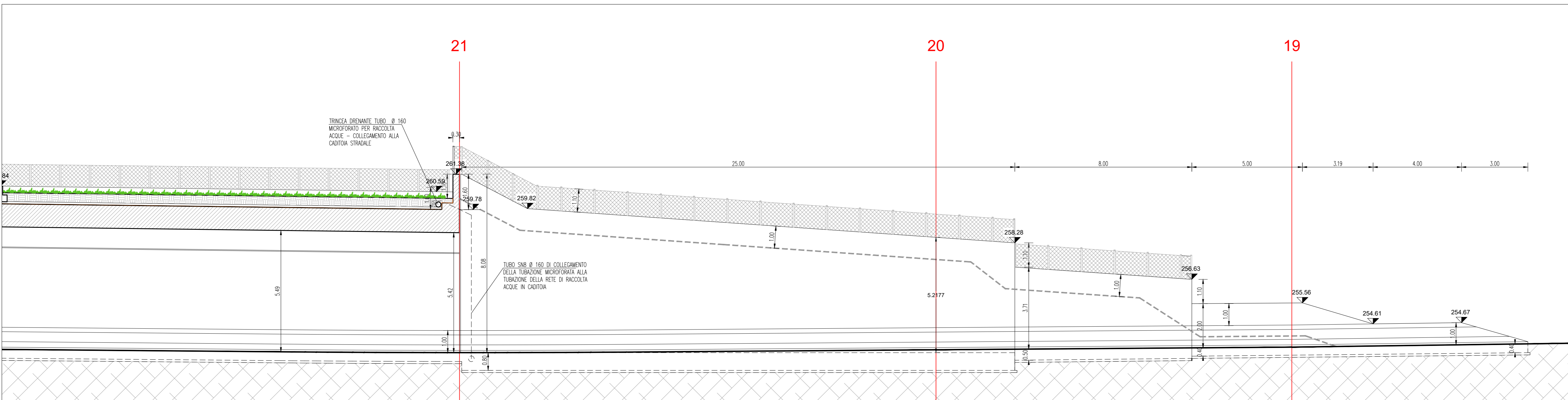
SEZIONE/PROSPETTO A_A - VISTA SUD - LATO SOLZA - Scala 1:100
