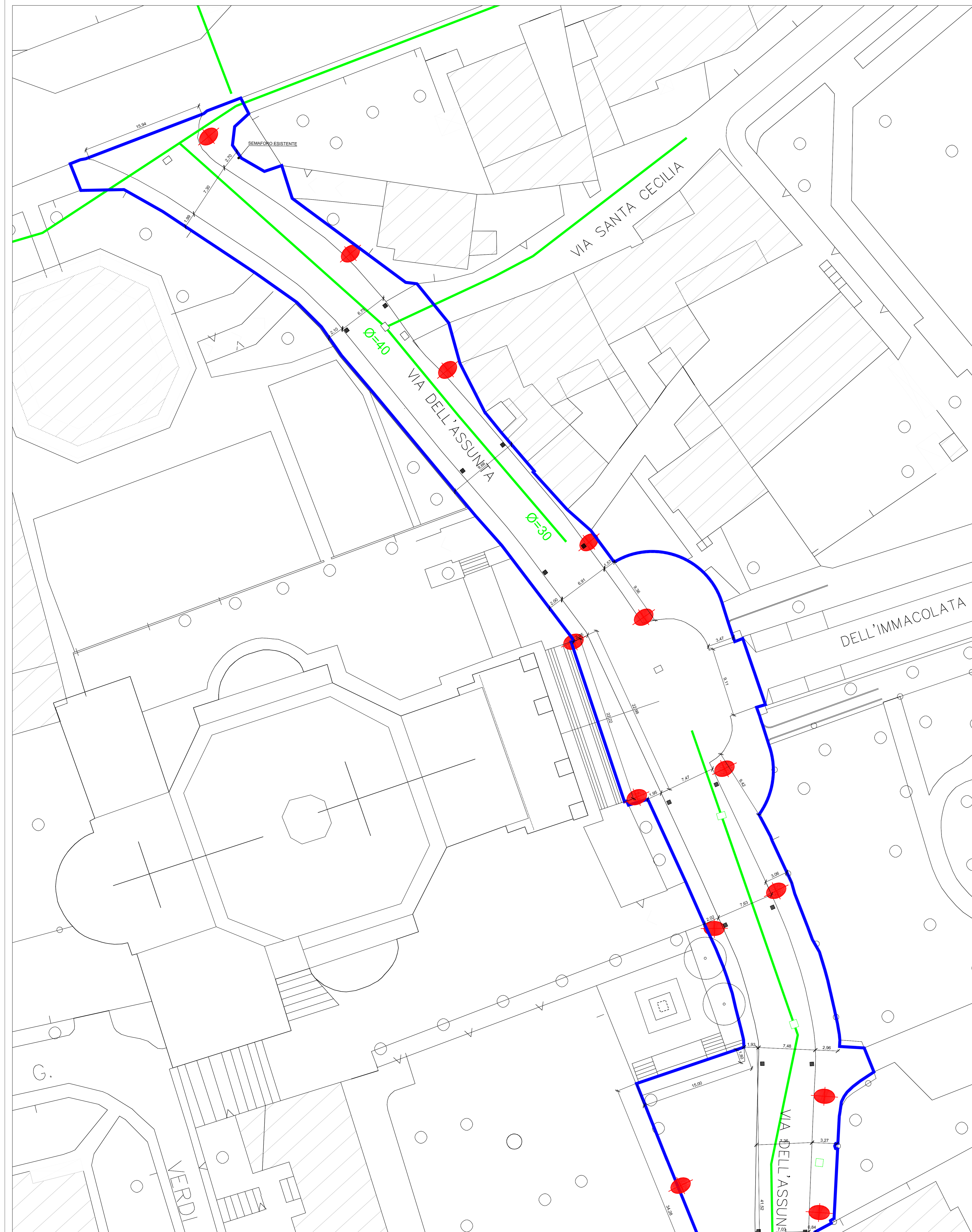
PLANIMETRIA GENERALE - STATO DI FATTO SCALA 1.200
