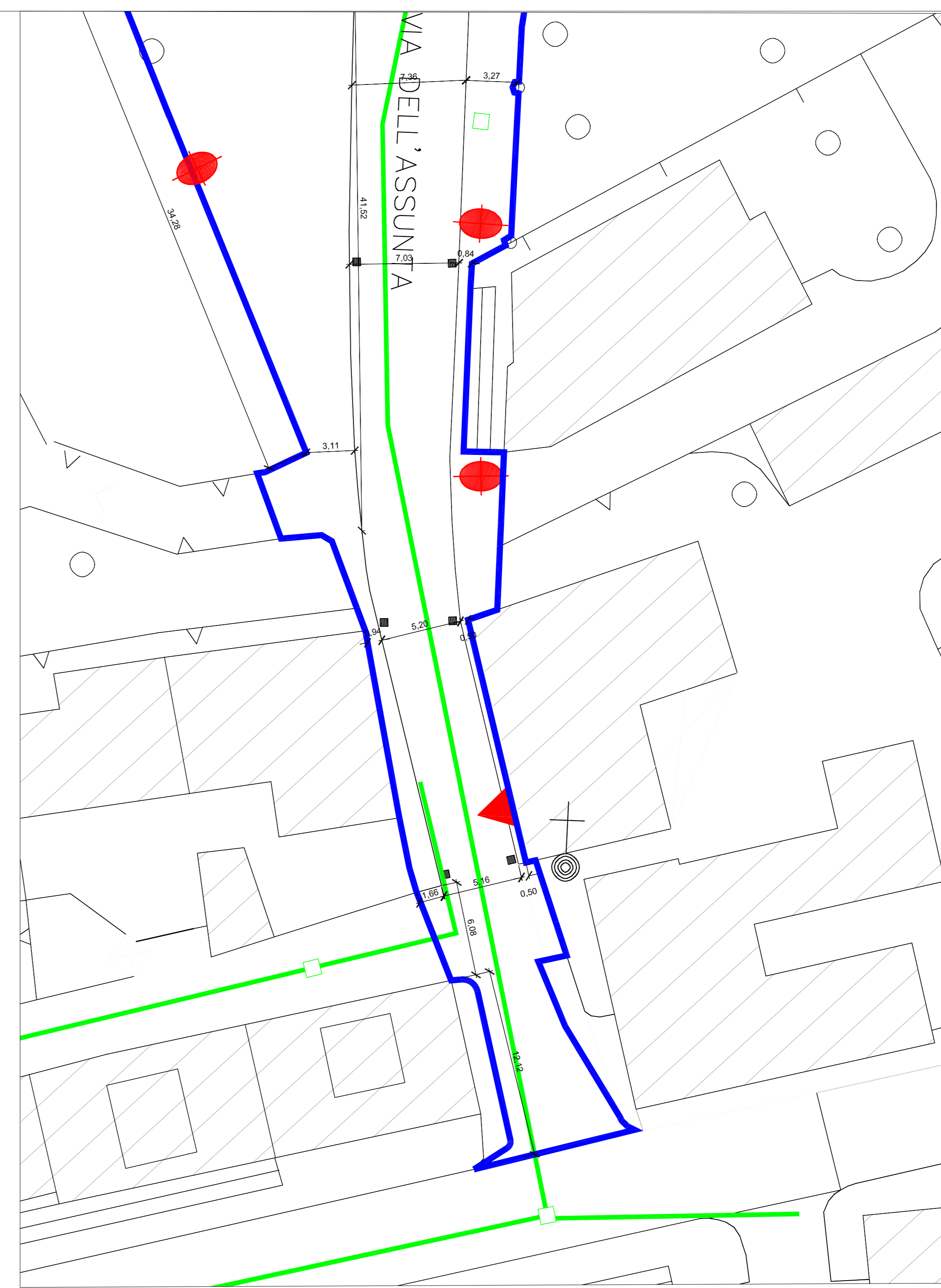
PLANIMETRIA GENERALE - STATO DI FATTO SCALA 1.200
