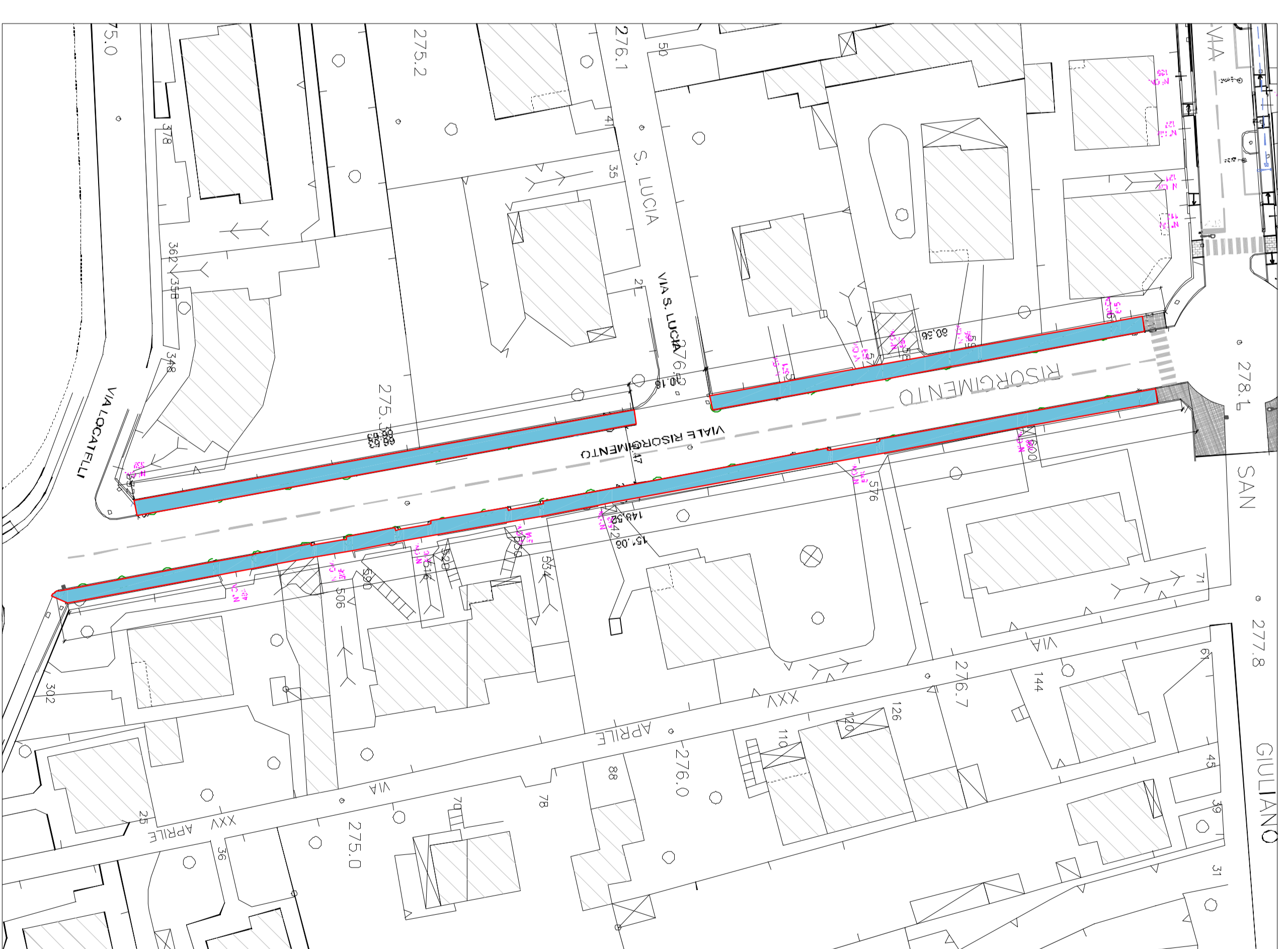
PROGETTO - PLANIMETRIA VIA RISORGIMENTO - SCALA 1:500
